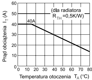
CHARAKTERYSTYKA OBCIĄŻALNOŚCI
