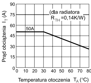
CHARAKTERYSTYKA OBCIĄŻALNOŚCI
