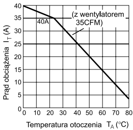
CHARAKTERYSTYKA OBCIĄŻALNOŚCI
